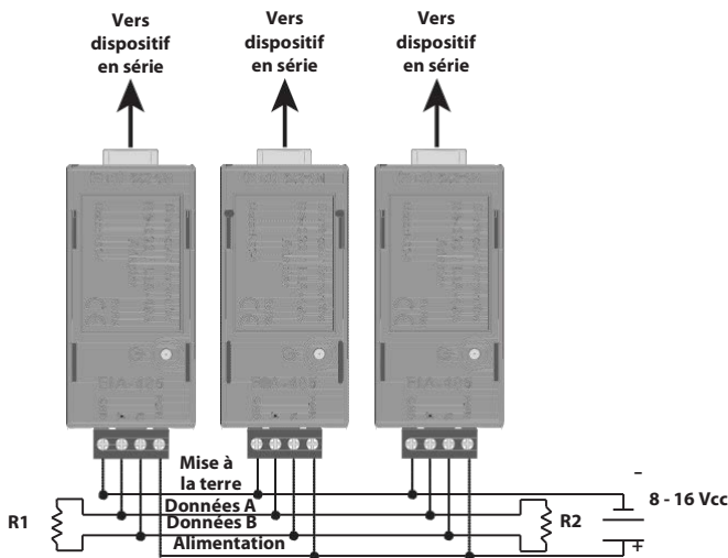
Figure 4. Câblage du bus EIA-485
