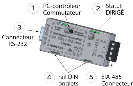
Figure 2. RSC-1, caractéristiques.
