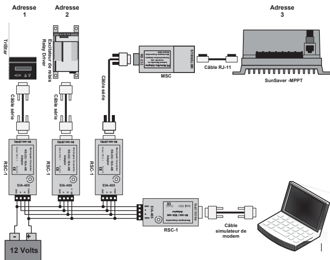
Figure 5. Exemple de réseau EIA-485 (résistances d'extrémité non illustrées)
