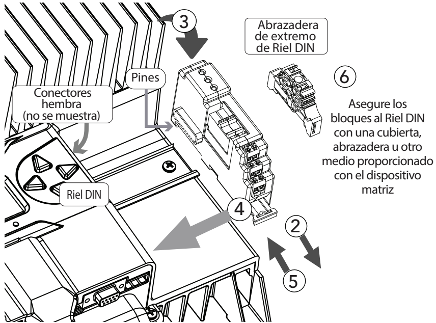
Figura 3-1. Detalle de instalación del ReadyRelay
