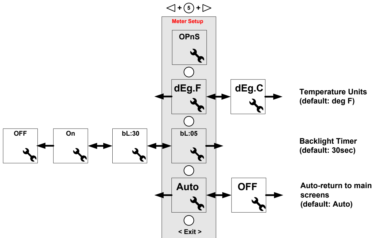
Abbildung 6: Anzeigeinstrument-Optionsmenü
