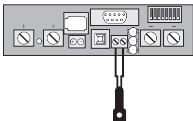
Abbildung 2.2 Anschluss des Temperatur-Fernfühlers
