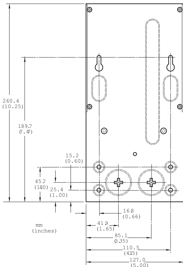
Figura 2.0 Dimensiones del montaje
